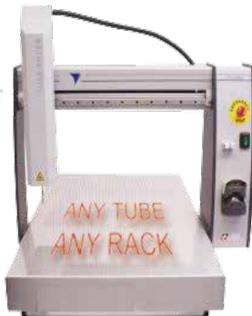
瑞士精密儀器 - 試管自動分注儀。
